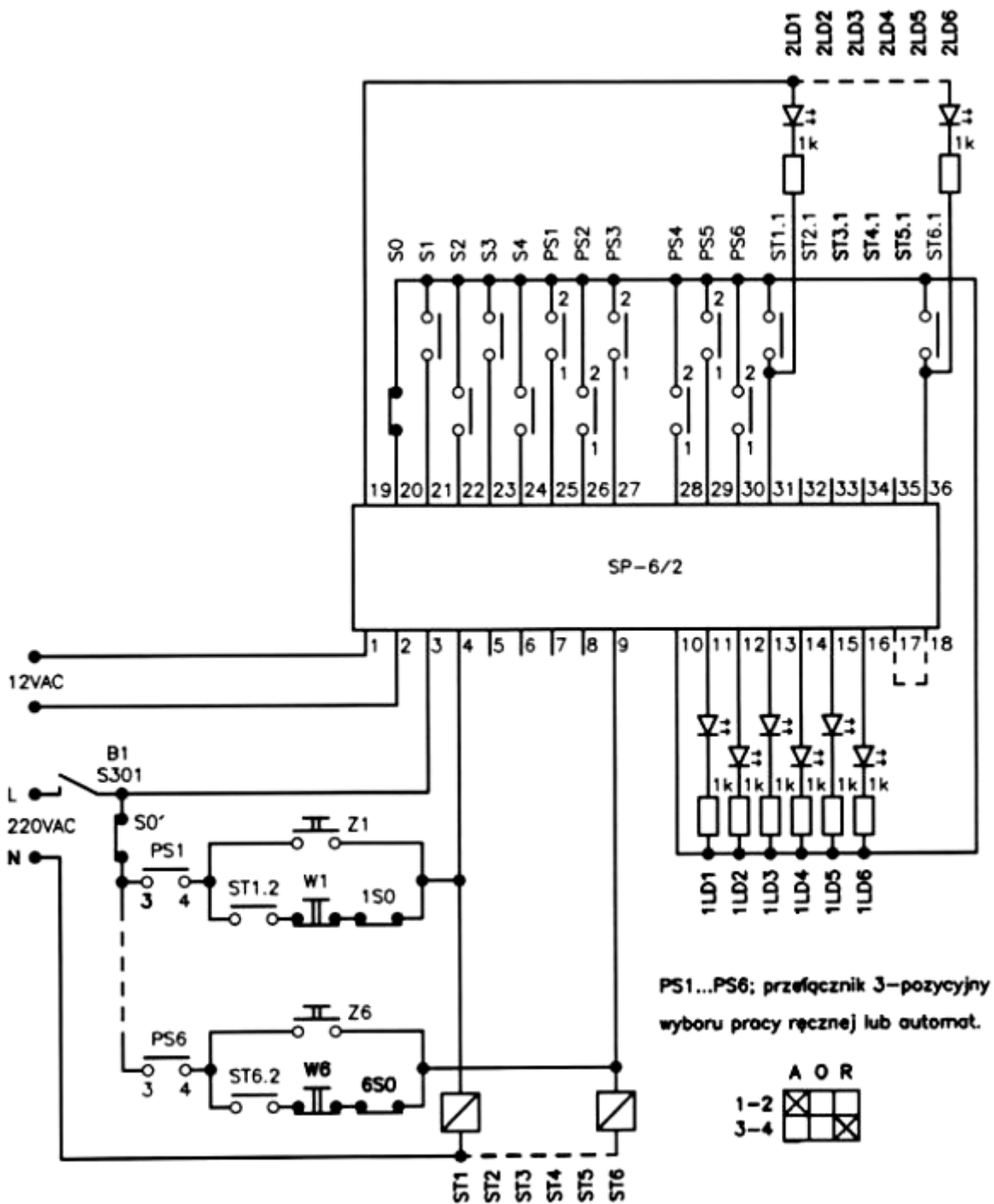
Rys. 2. Aplikacja podłączenia sterownika SP-6/2 w układ sterowania sześciu pomp sterowanych czterema czujnikami (poziomu ,ciśnienia)
