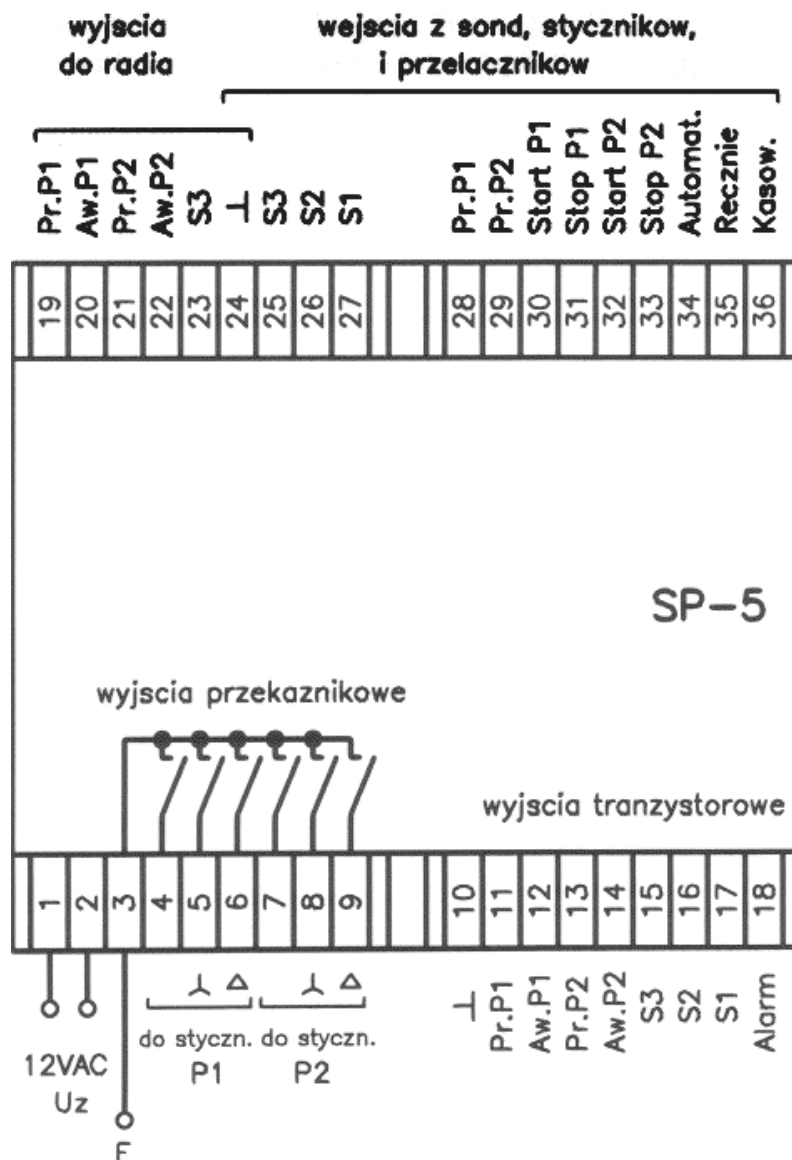
Rys.2 Sposób podłączenia sterownika SP-5
