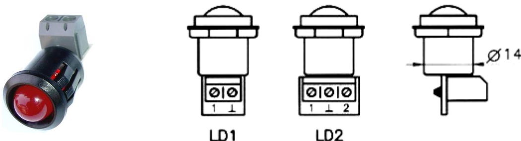
Rys. 5. Oprawki z diodami typu LD1 i LD2 do zewnętrznej sygnalizacji optycznej
