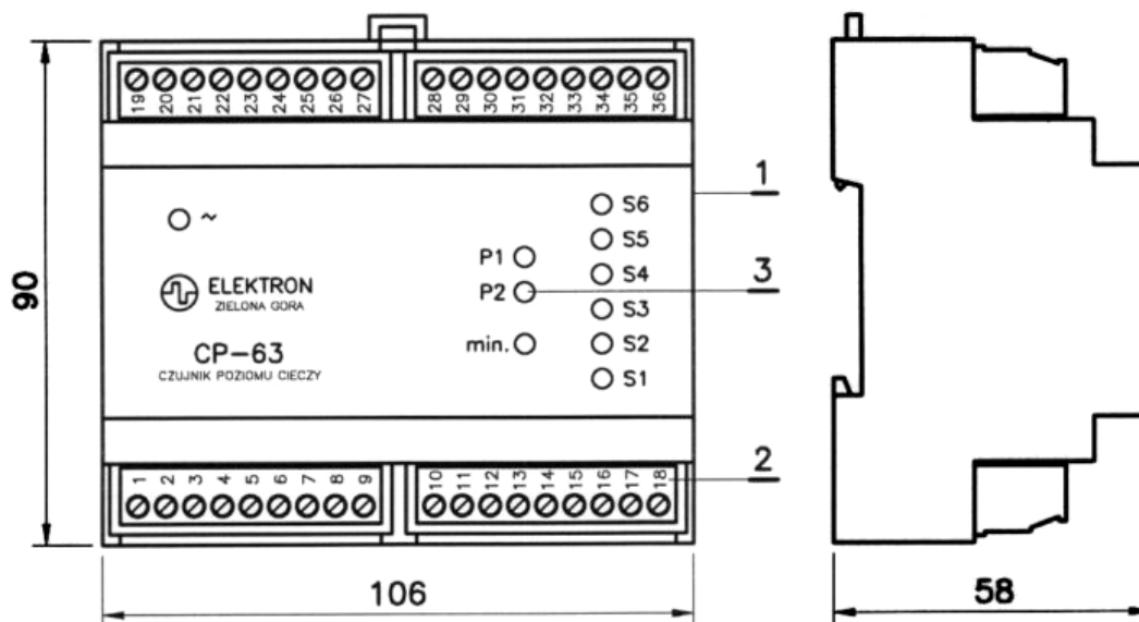
Rys. 1 Obudowa czujnika CP-63 z widokiem płyty czołowej.
