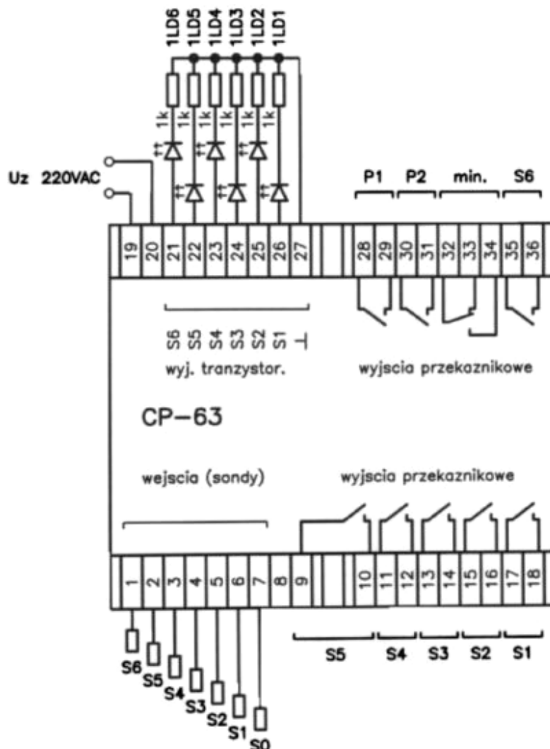
Rys.2. Schemat podłączenia czujnika CP-63.
