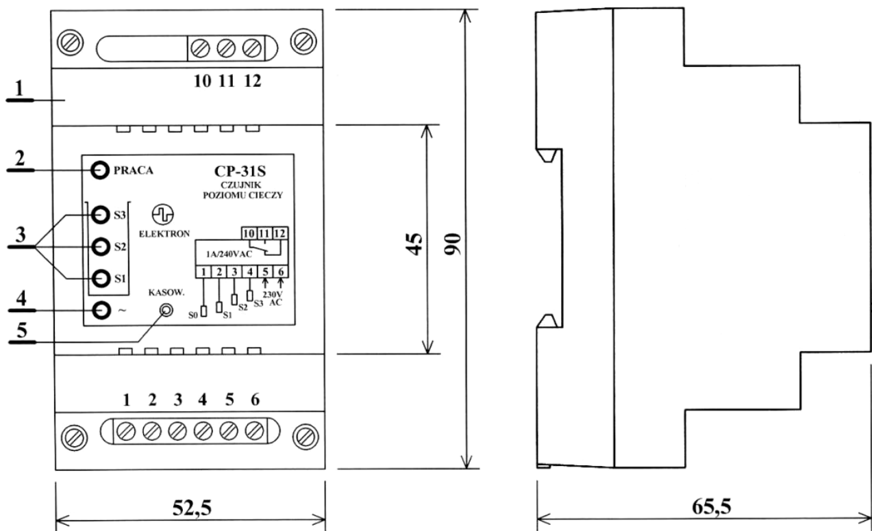
Rys. 1 Obudowa czujnika CP-31S z widokiem płyty czołowej.
