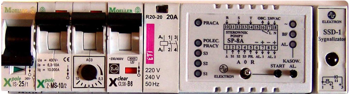
Rys. 2. Zespół sterowania pompy (przykład)
