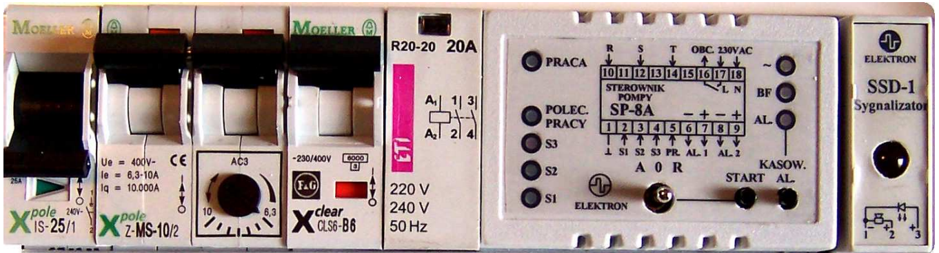
Rys. 1. Zespół sterowania pompy ( przykład)
