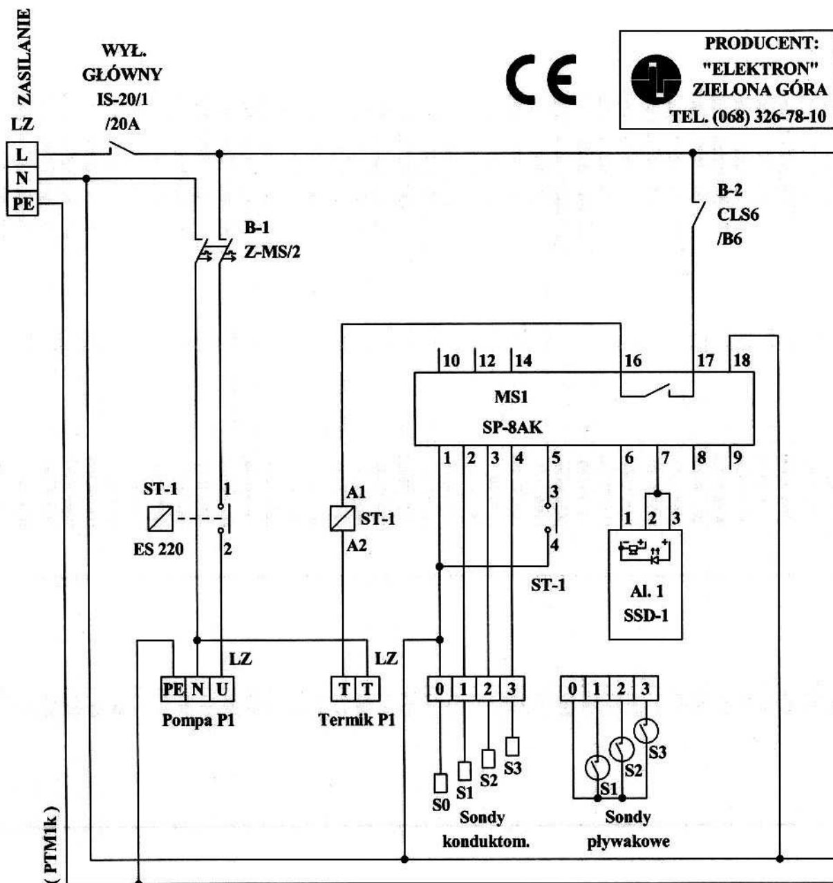
Rys. 3. Przykładowy schemat sterowania pompy 1-fazowej z zastosowaniem sterownika „SP-8AK” Przy zastosowaniu sterownika „SP-8A” – sondy tylko w wersji pływakowej.
