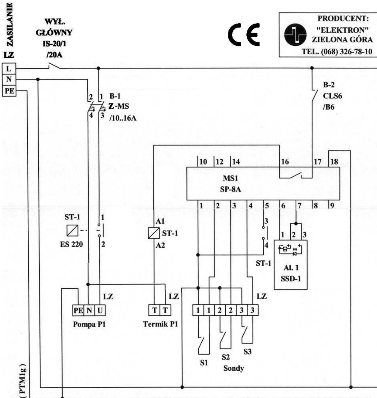
Rys. 3. Przykładowy schemat sterowania pompy 1-fazowej z zastosowaniem sterownika „SP-8A”
