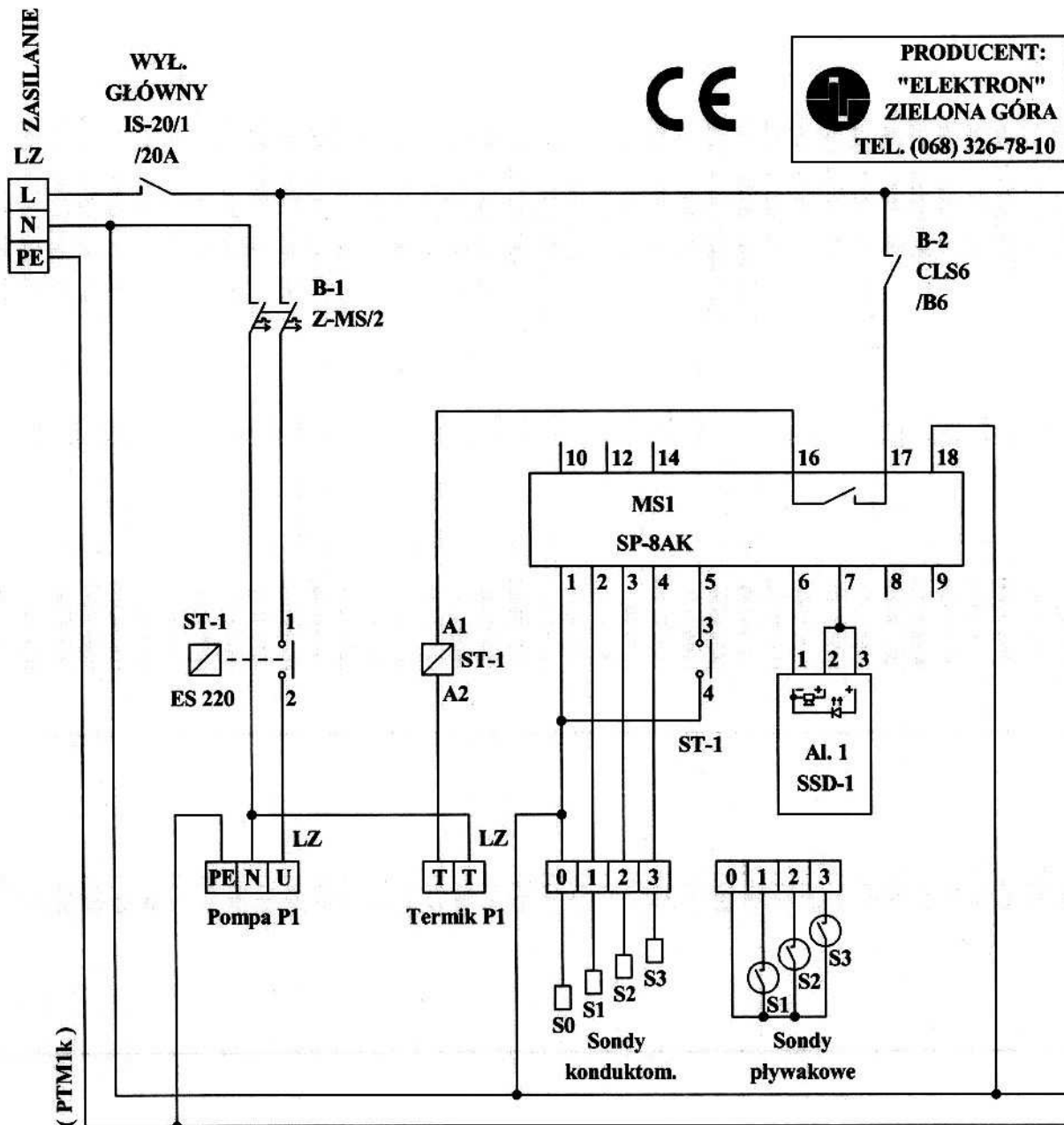
Rys. 2. Przykładowy schemat sterowania pompy 1-fazowej z zastosowaniem sterownika „SP-8AK” Przy zastosowaniu sterownika „SP-8A” – sondy tylko w wersji pływakowej.
