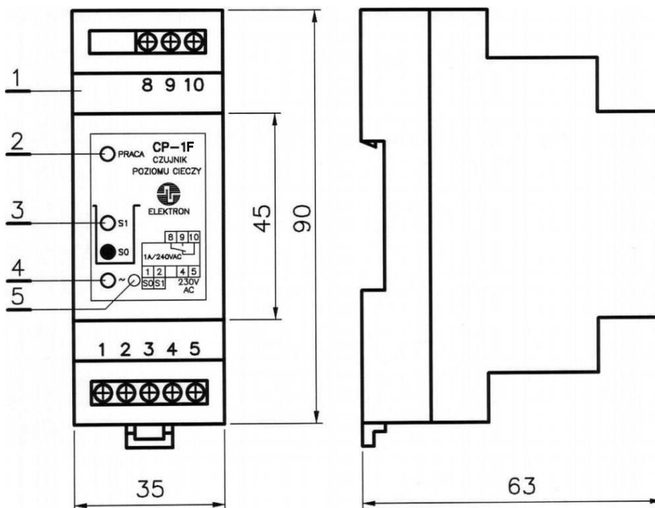
Rys. 1 Obudowa czujnika CP-1F z widokiem płyty czołowej.
